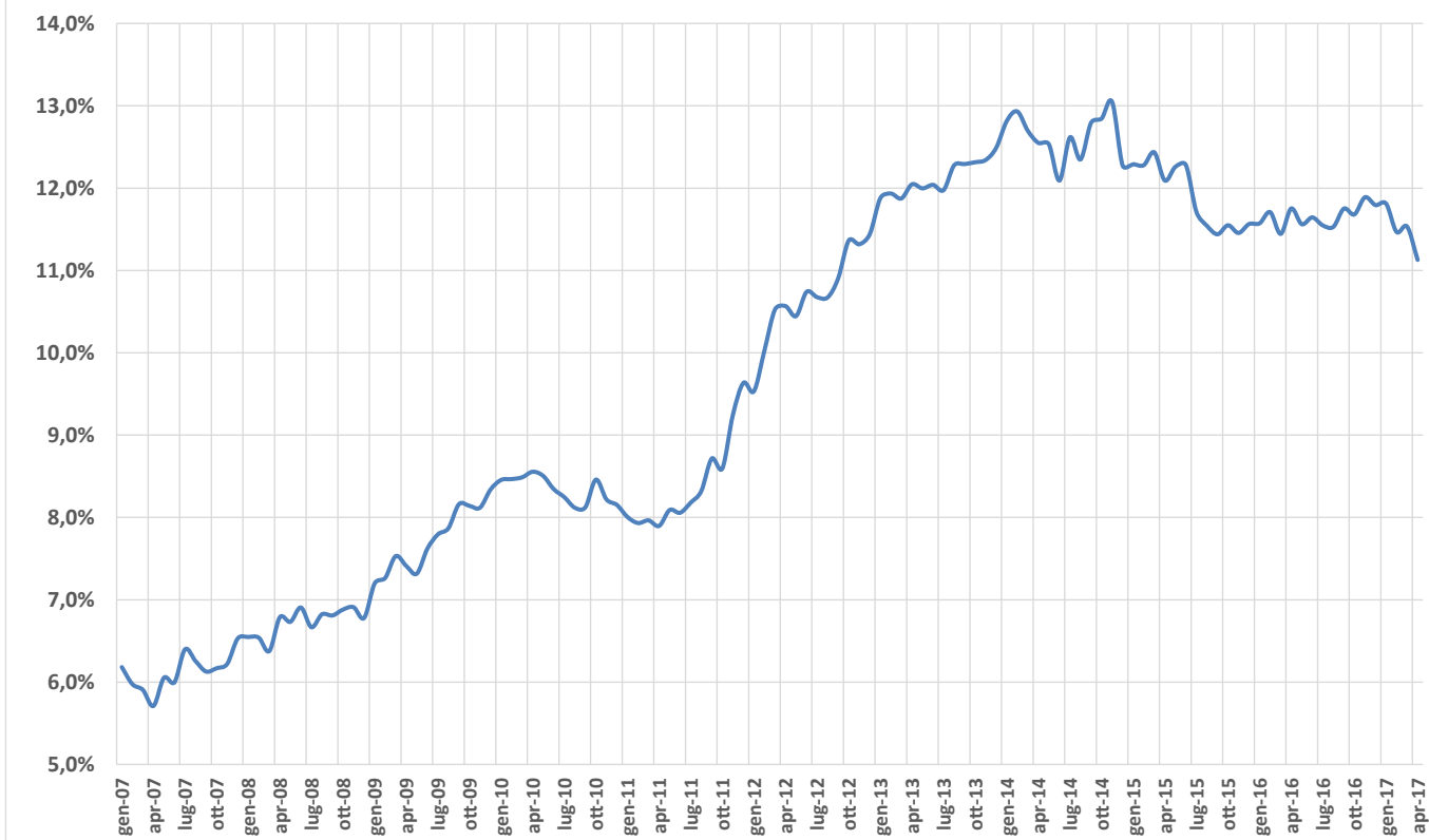
Tasso di disoccupazione gennaio 2007 - aprile 2017
