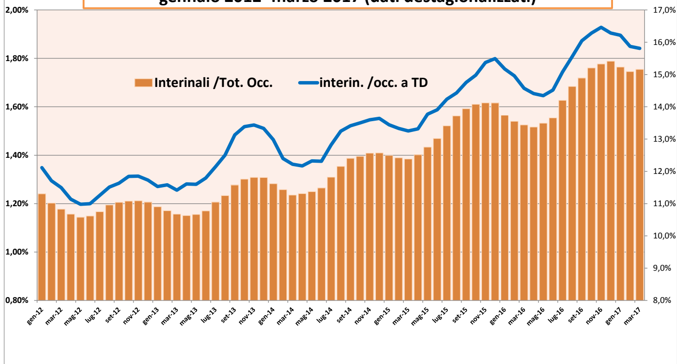
Fig. 8 Quota dell'occupazione interinale sul totale e sull'occupazione a tempo determinato (scala destra), gennaio 2012- marzo 2017 (dati destagionalizzati)
